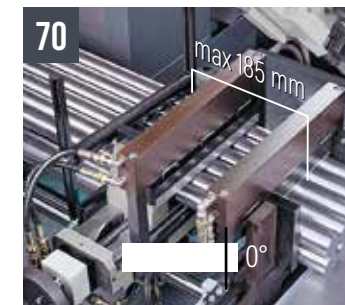
70 SHARK 331-1 NC 5.0 spider - Étaux verticaux hydrauliques pour coupe en paquets (max 320x150 mm)
