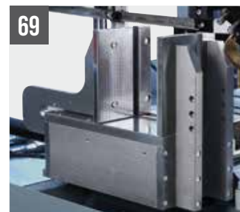
69 SHARK 230-1 NC HS 5.0 étau de coupe à double serrage
